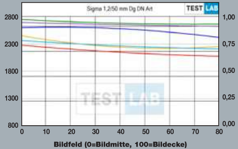
Auflösung (LP/BH) Kontrast
