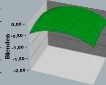
Vignettierung - Blende offen
